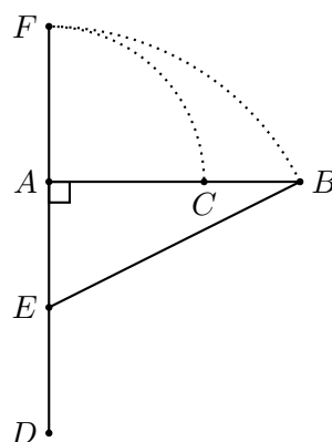
Figura 1: Separación áurea con regla y compás
