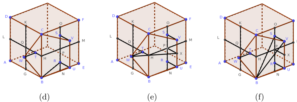
Figura 5: Construcción del dodecaedro: la métrica
