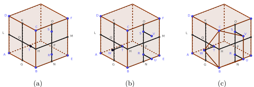
Figura 4: Construcción del dodecaedro: las caras
